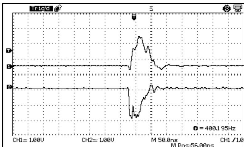
Rys.2. Zobrazowanie przebiegów impulsu nadawczego (dolny) oraz impulsu odwróconego (górny) podawanego na wejście wyzwalające generatora sygnałowego.
