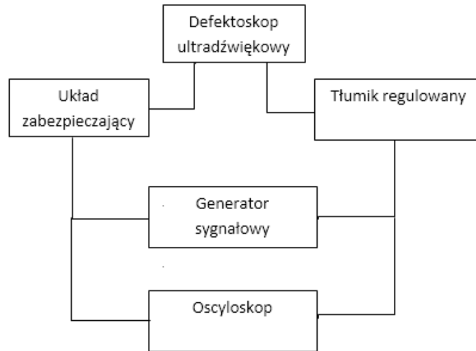
Rys.1. Schemat połączeniowy układu do testowania defektoskopu ultradźwiękowego.
