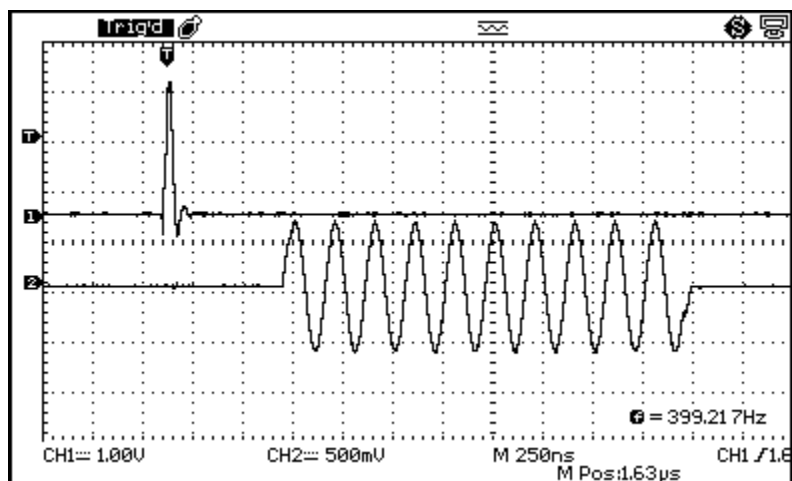
Rys 3. Przebiegi typowych sygnałów z nadajnika defektoskopu (górny) oraz sygnału testowego z generatora sygnałowego (dolny).
