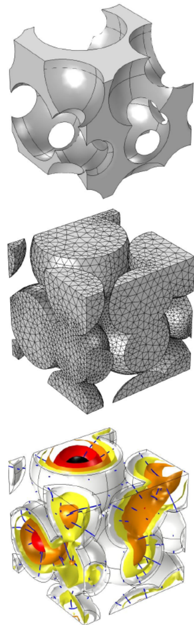
Rys.: Reprezentatywny Element Objętościowy dla pianki o porowatości otwartej 70%: periodyczny szkielet, siatka elementów skończonych na obszarze płynu w porach oraz wyniki obliczeń numerycznych na poziomie mikro-skali.
