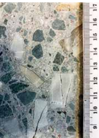
Fot. 4. Przekrój odwiertu betonowego z widocznymi spękaniami ziaren kruszywa (ale tylko jasnoszarych, ziarna ciemnoszare nie-spękałe)
