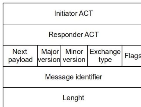
Fig. 2. ISAKMP header
