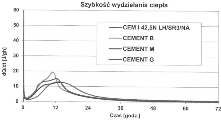
Rys. 2. Szybkość wydzielonego ciepła cementów z proszkowym dodatkiem minerałów ciężkich
