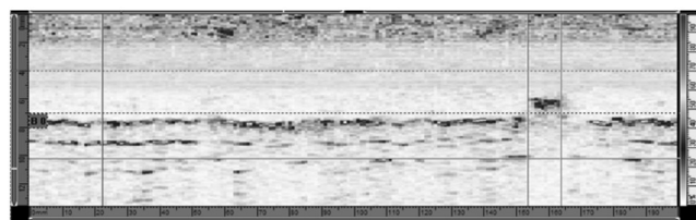
Rys. 11. Zobrazowanie typu B obrazujące wadę typu brak przetopu (między czerwonym i zielonym kursorem) na tle echa kształtu od wycieku z grani
