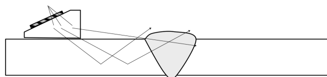
Rys. 1. Skanowanie ustalonymi kątami wiązek (rastrowe lub wzdłuż spoiny)
