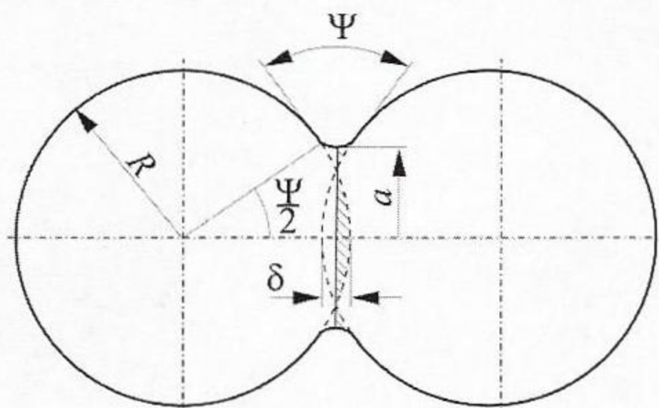
Fig. 3. Model parameters definition
